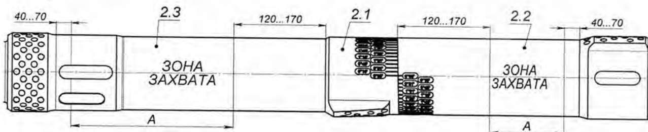
Рисунок 3 (Меньшие значения размеров для ВЗД габаритов 106 мм и менее)
