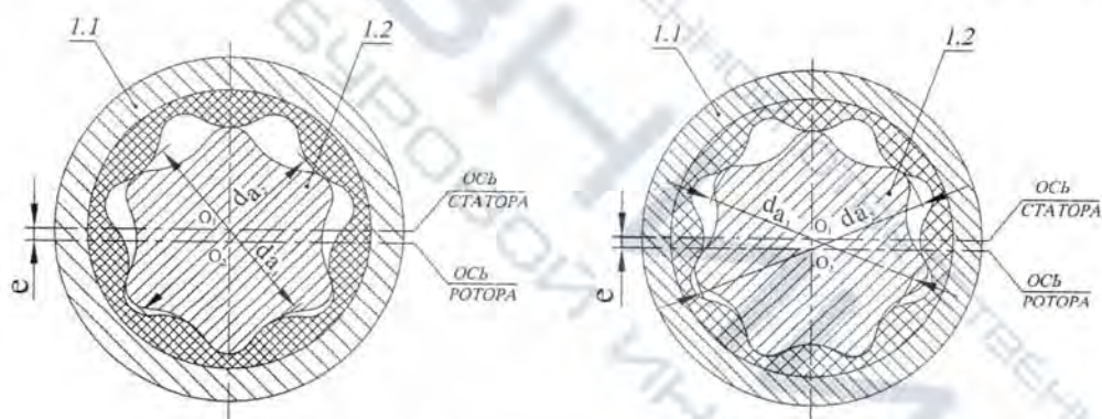
Ротор с нечетным количеством зубьев
